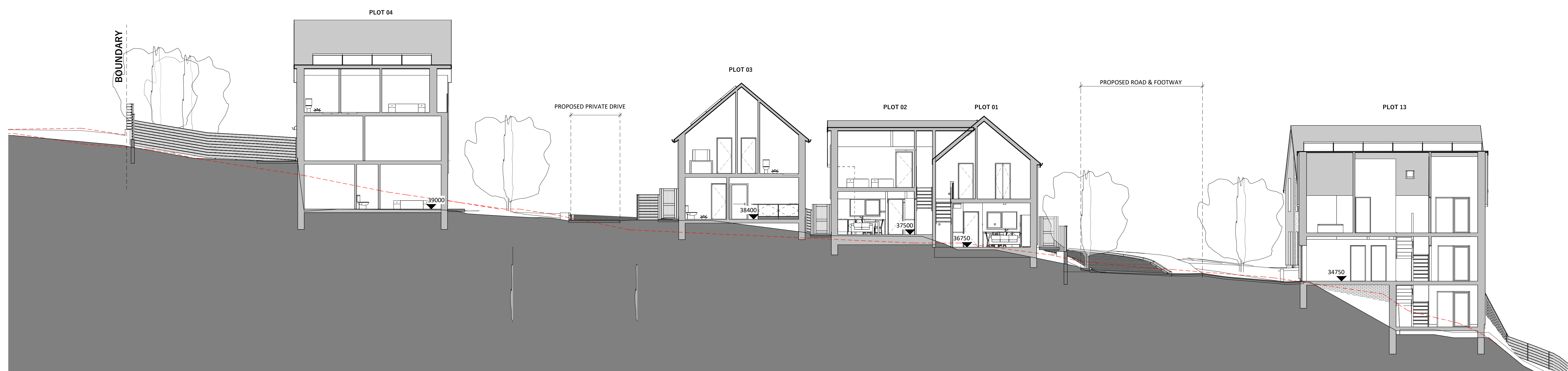
SECTION 01 SCALE: 1:100
