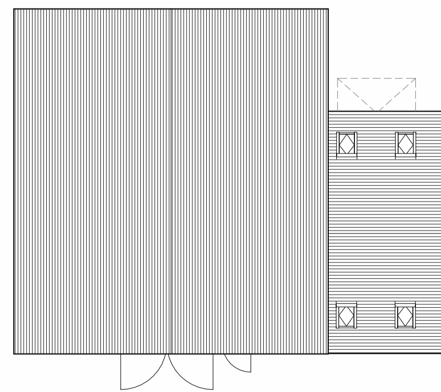
03 - ROOF SCALE: 1 : 100
