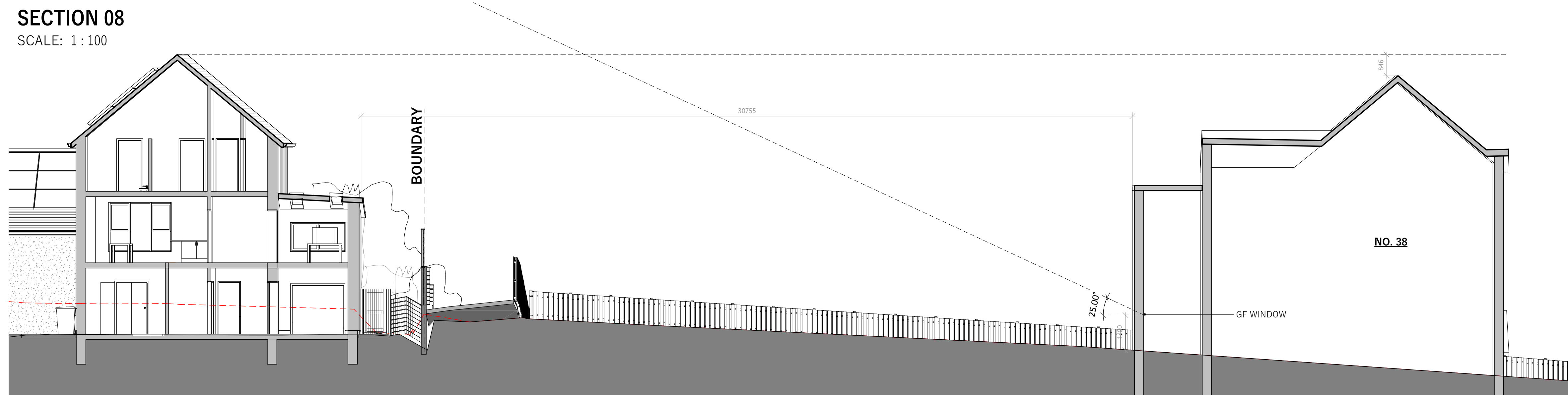
SECTION 09 SCALE: 1 : 100
